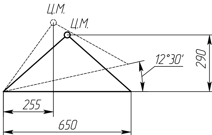
Рисунок 1- Схема устойчивости агрегата типа 1КсВ
